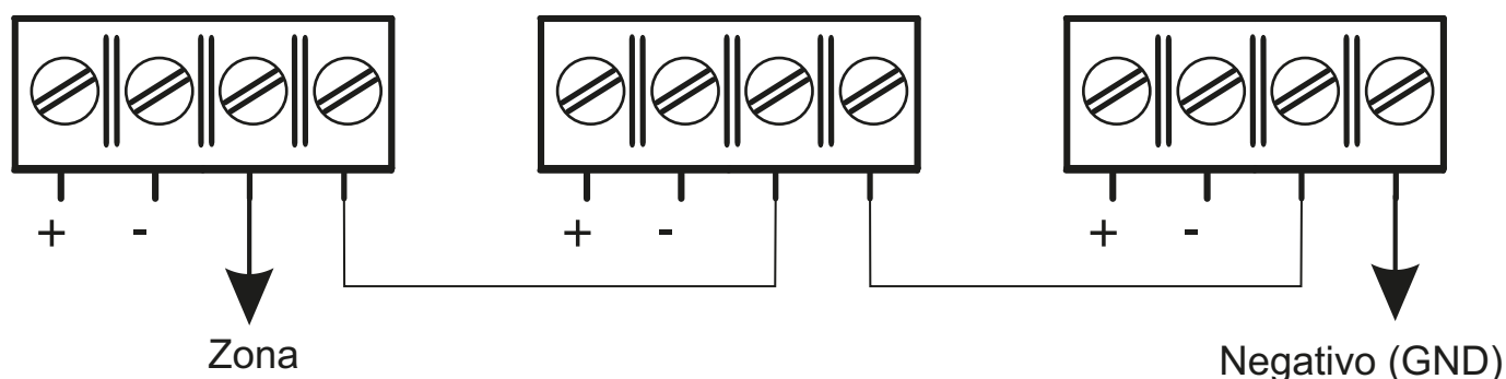
FIG. 3: Ligação em Série
